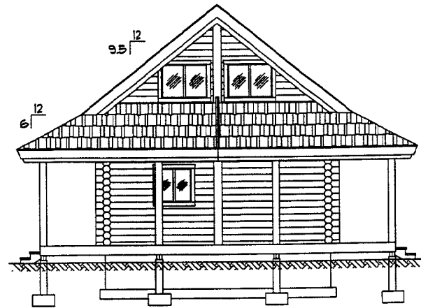
RIGHT ELEVATION
